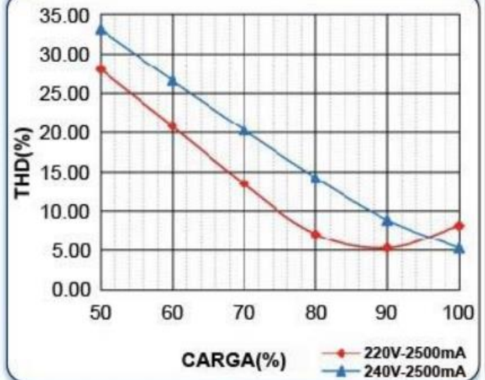
Distorsión armónica Vs Carga
